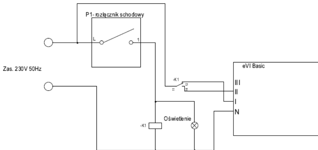
Rys. E.3: Podłączenie dwubiegowe + oświetlenie
