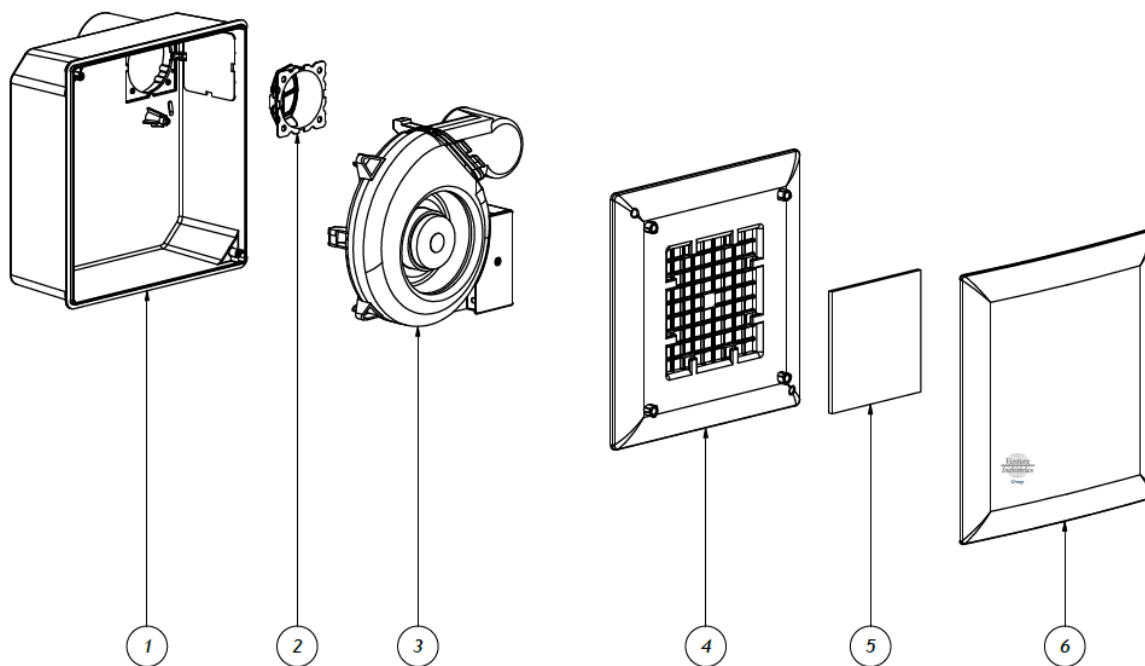
Rys. 2.3: Budowa wentylatora eVI EC R T
