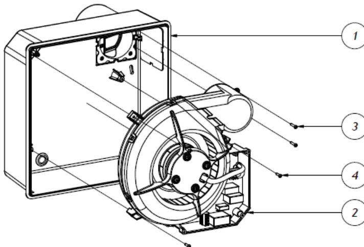
Rys. 4.11: Montaż wentylatora w obudowie
