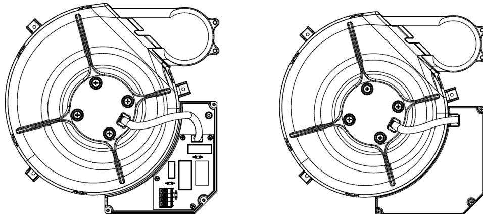
Rys. 4.14: Pokrywa elektryczna eVI
