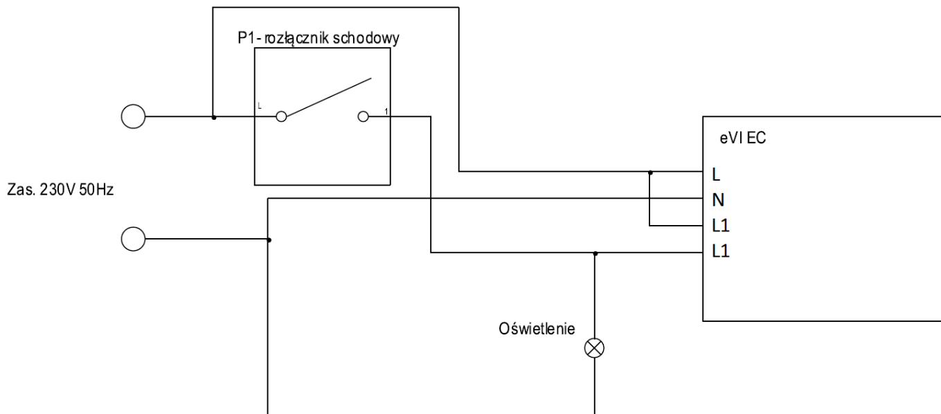
Rys. E.8: Podłączenie dwubiegowe + oświetlenie
