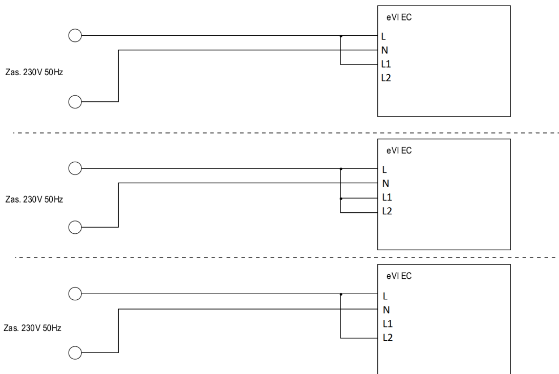
Rys. E.6: Podłączenie jednobiegowe
