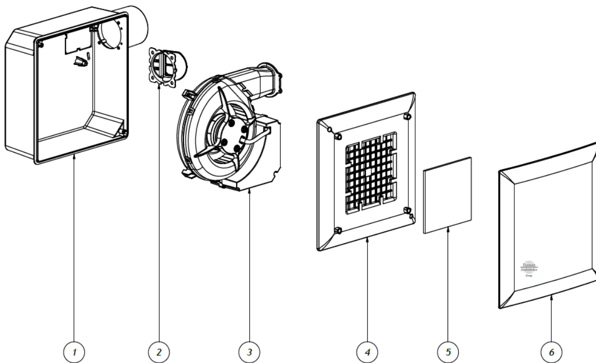
Rys. 2.2: Budowa wentylatora eVI S
