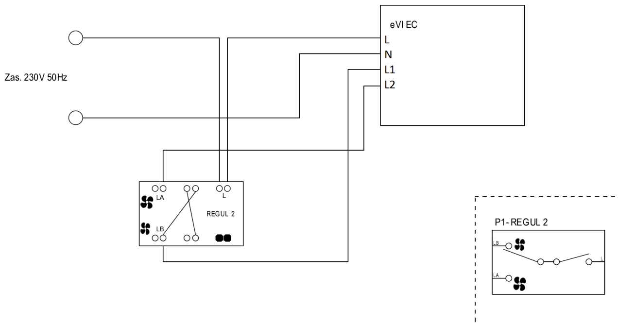
Rys. E.7: Podłączenie dwubiegowe
