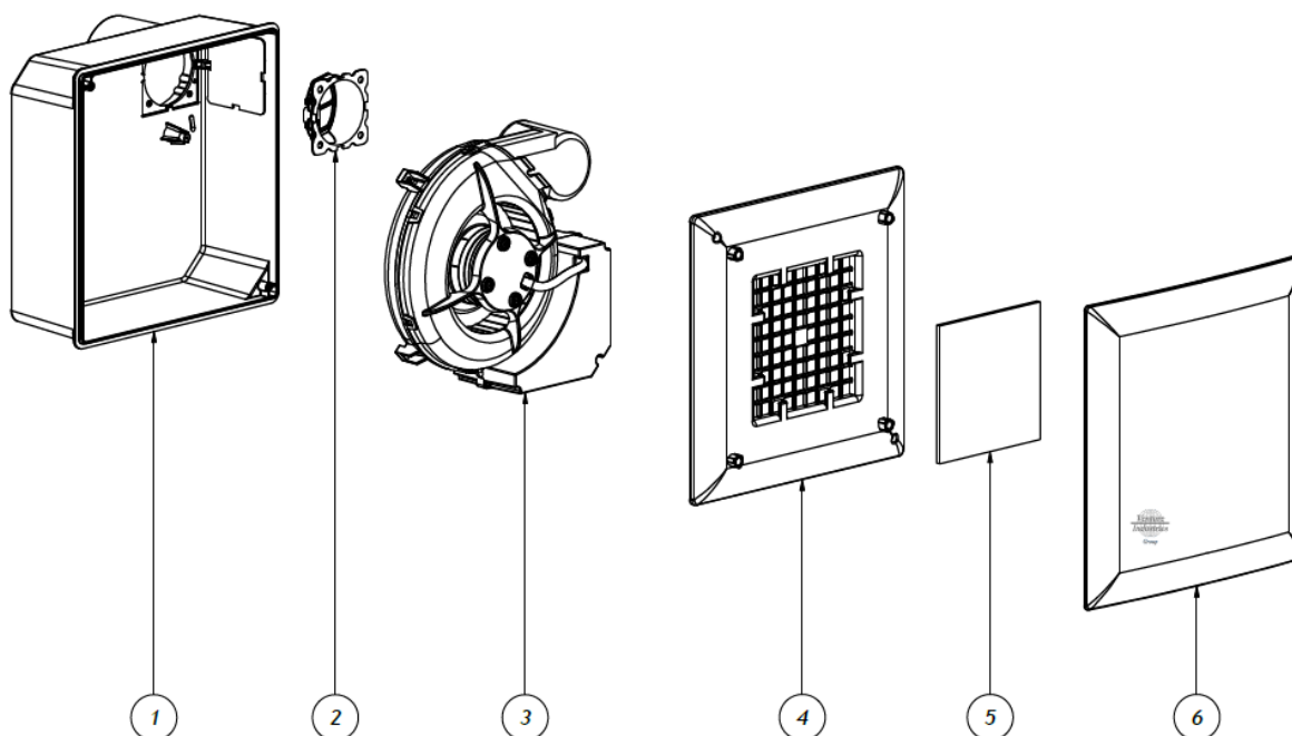
Rys. 2.1: Budowa wentylatora eVI R
