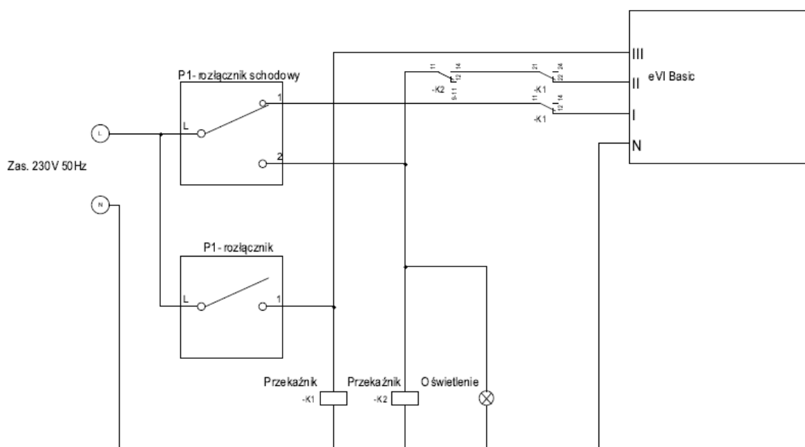
Rys. E.5: Podłączenie trójbiegowe + oświetlenie
