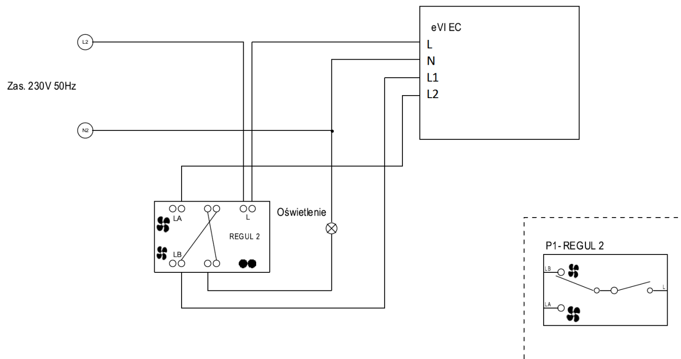
Rys. E.9 Podłączenie dwubiegowe + off + oświetlenie
