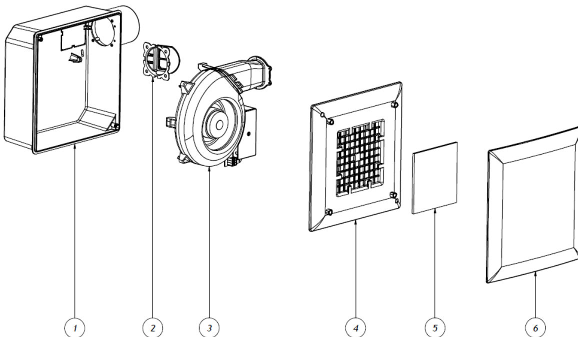
Rys. 2.4: Budowa wentylatora eVI EC S T
