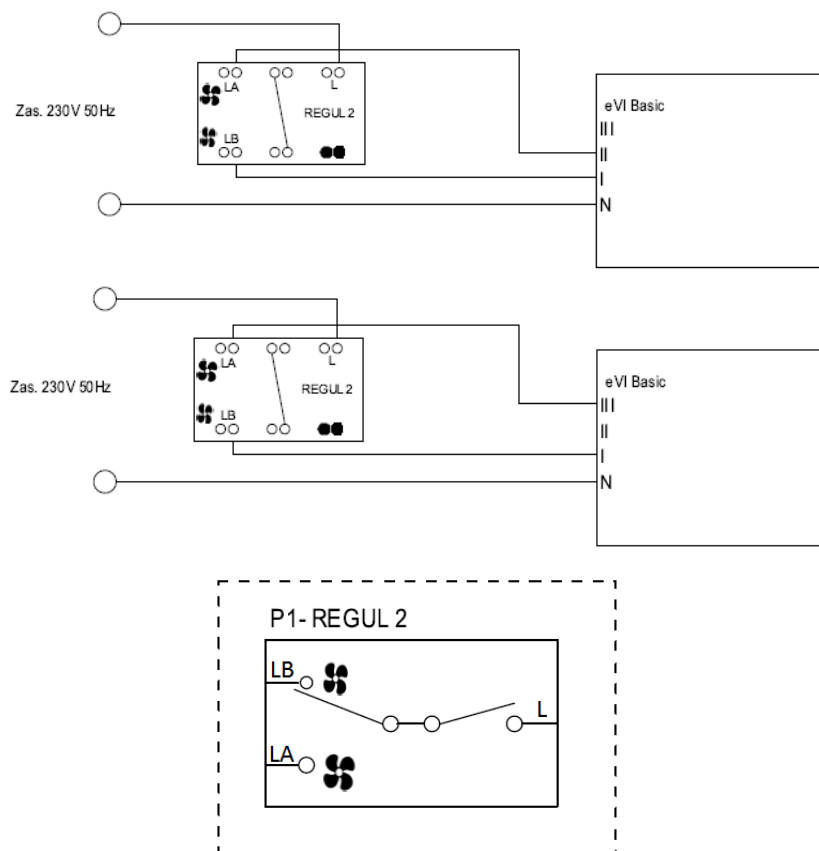
Rys. E.2: Podłączenie dwubiegowe
