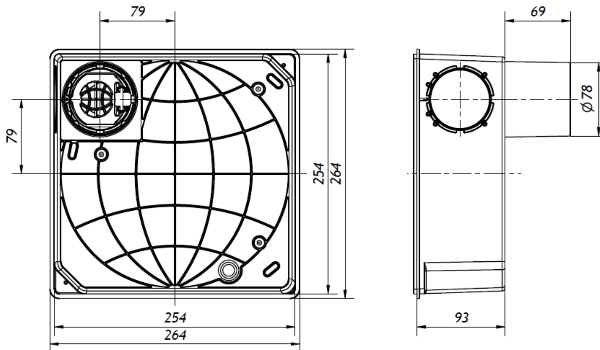
Rys. 4.1: eVI R, eVI EC R T – wymiary
