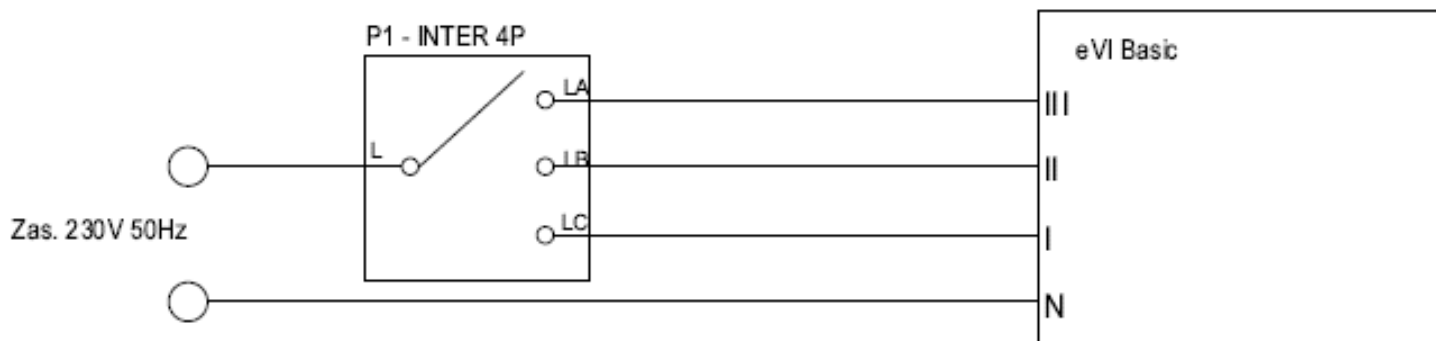
Rys. E.4: Podłączenie trójbiegowe
