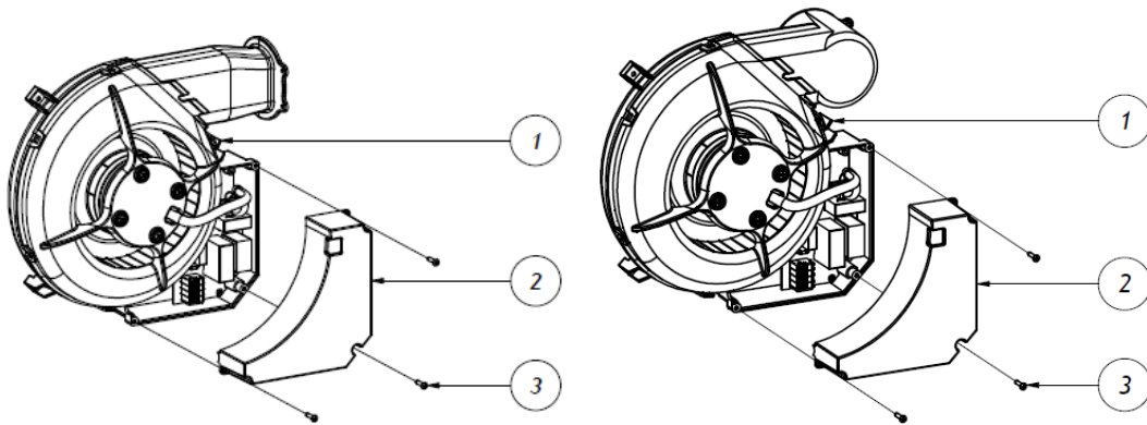
Rys. 4.13: Pokrywa elektryczna eVI
