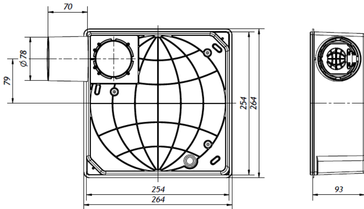
Rys. 4.2: eVI S, eVI EC S T - wymiary
